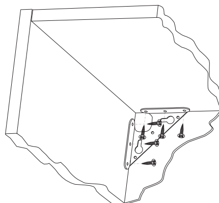
6 TORNILLOS 072433 (4x20mm)
