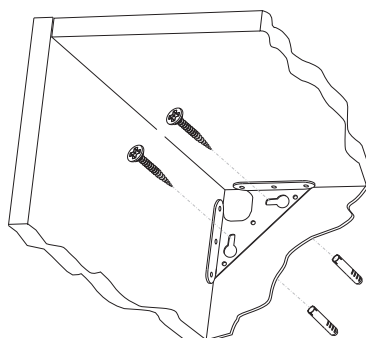
2 TACOS DE NYLON 079010 A LA PARED Y 2 TORNILLOS 072456 (5x40mm)
